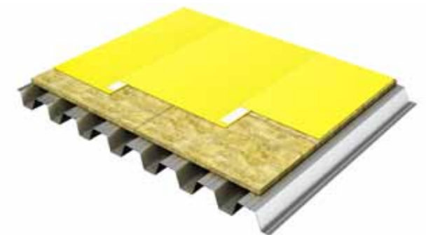
14 pav. Garų izoliacijos sluoksnio įrengimas ant profiliuoto lakšto
