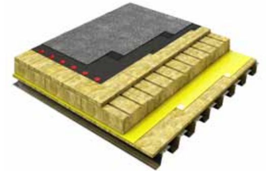
10 pav. Konstrukcija iš dviejų sluoksnių mineralinės šilumos izoliacijos
