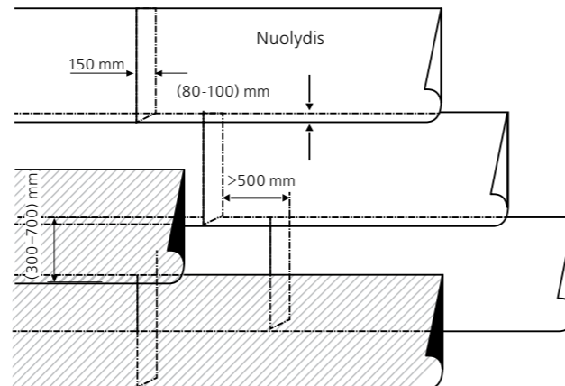
3 pav. Poslinkis sutampančiuose stogo dangų sluoksniuose
