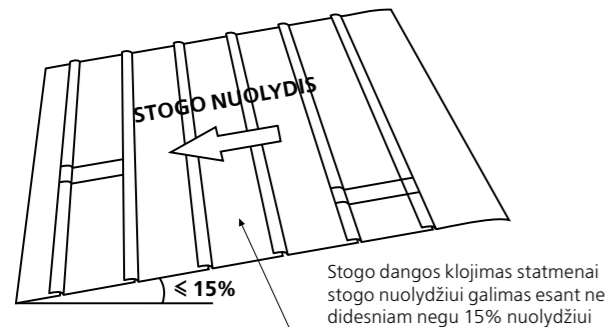
1 pav. Dengimas danga ant šlaito
