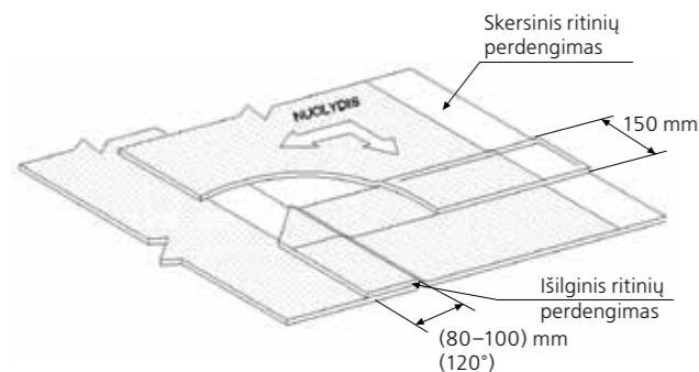
2 pav. Ritinių dangų perdengimas tvirtinant medžagas mechanškai
